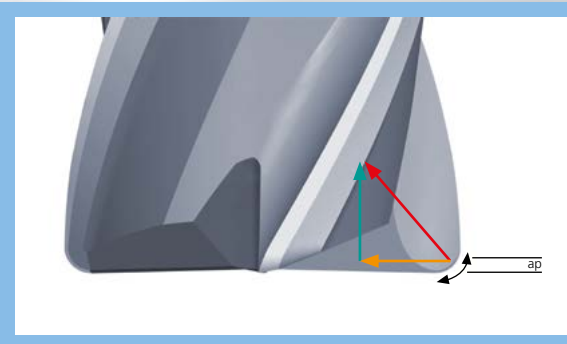
Sarokrádiuszos szerszám
